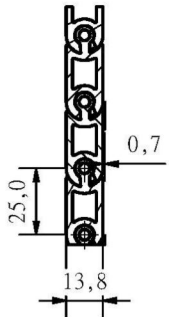
B-B (1:2)
